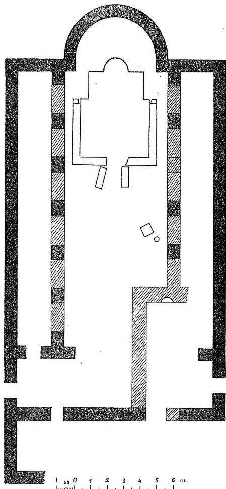
Сл. 3. — Основа старохришћанске базилике (стање после ископавања 1931 год.).
